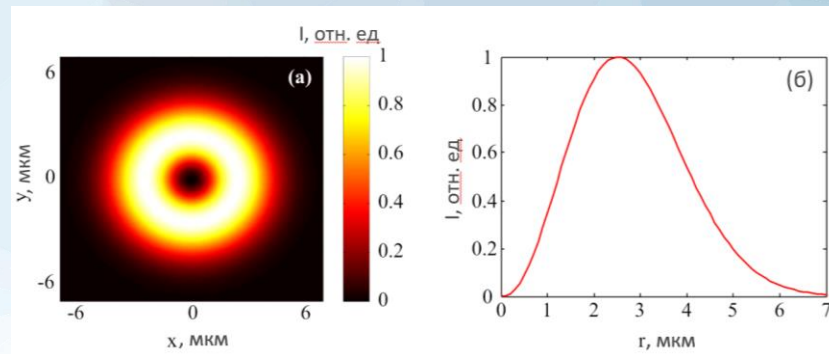
Рис. 3. Входной радиально поляризованный свет с перетяжкой \delta = 0,5 \mu\text{м} : распределение в плоскости XY (а) и по радиусу r (б).
